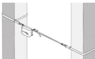
2. Ancoragem Temporal
